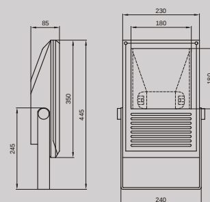
HQI-150
